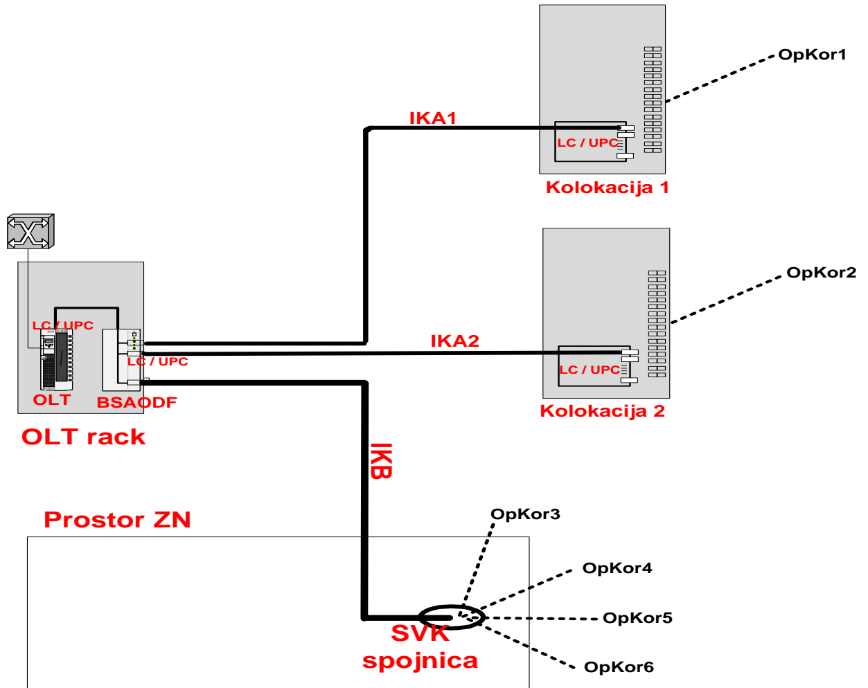
Slika 1. Načini spajanja svjetlovodnog provodnog kabla Operatora korisnika na ODF HT-a
