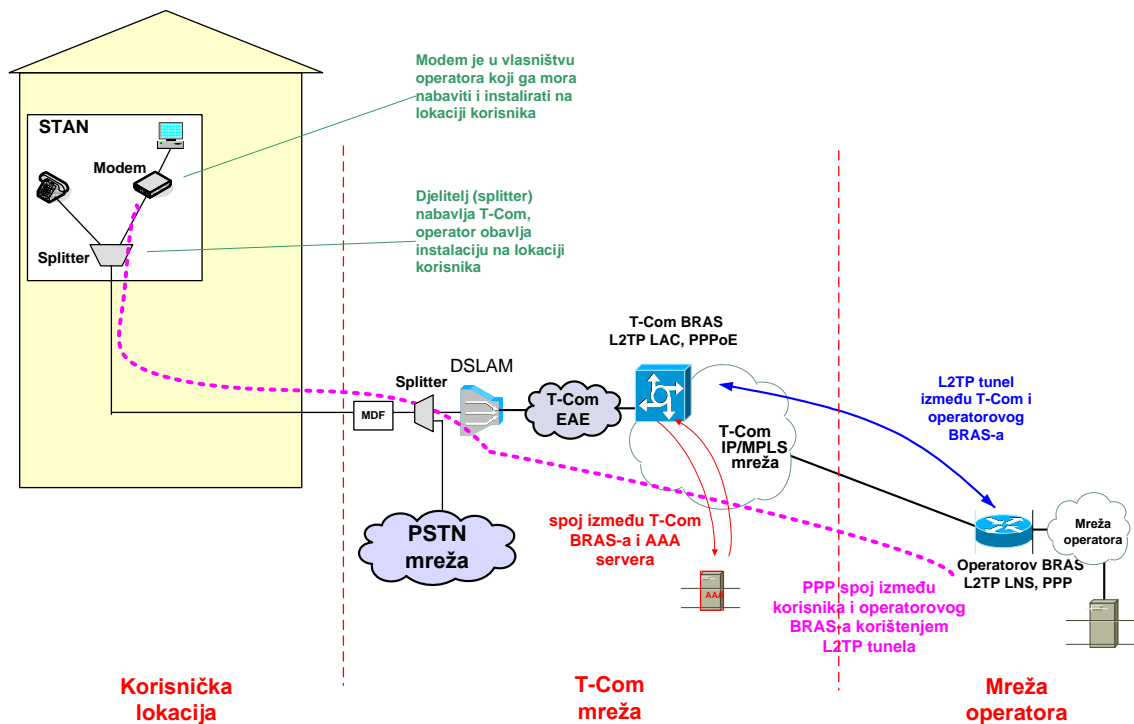
Slika 1. Način realizacije usluge veleprodajnog širokopolasnog pristupa za Internet uslugu korištenjem ADSL/VDSL tehnologije na IP razini
