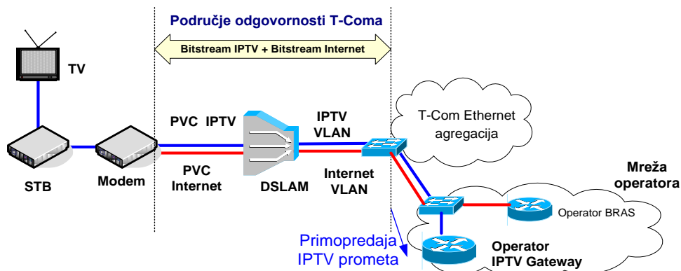
Slika 27. Veleprodajni širokopoljasni pristup za pružanje IPTV usluge preko ADSL/VDSL pristupa na DSLAM razini
